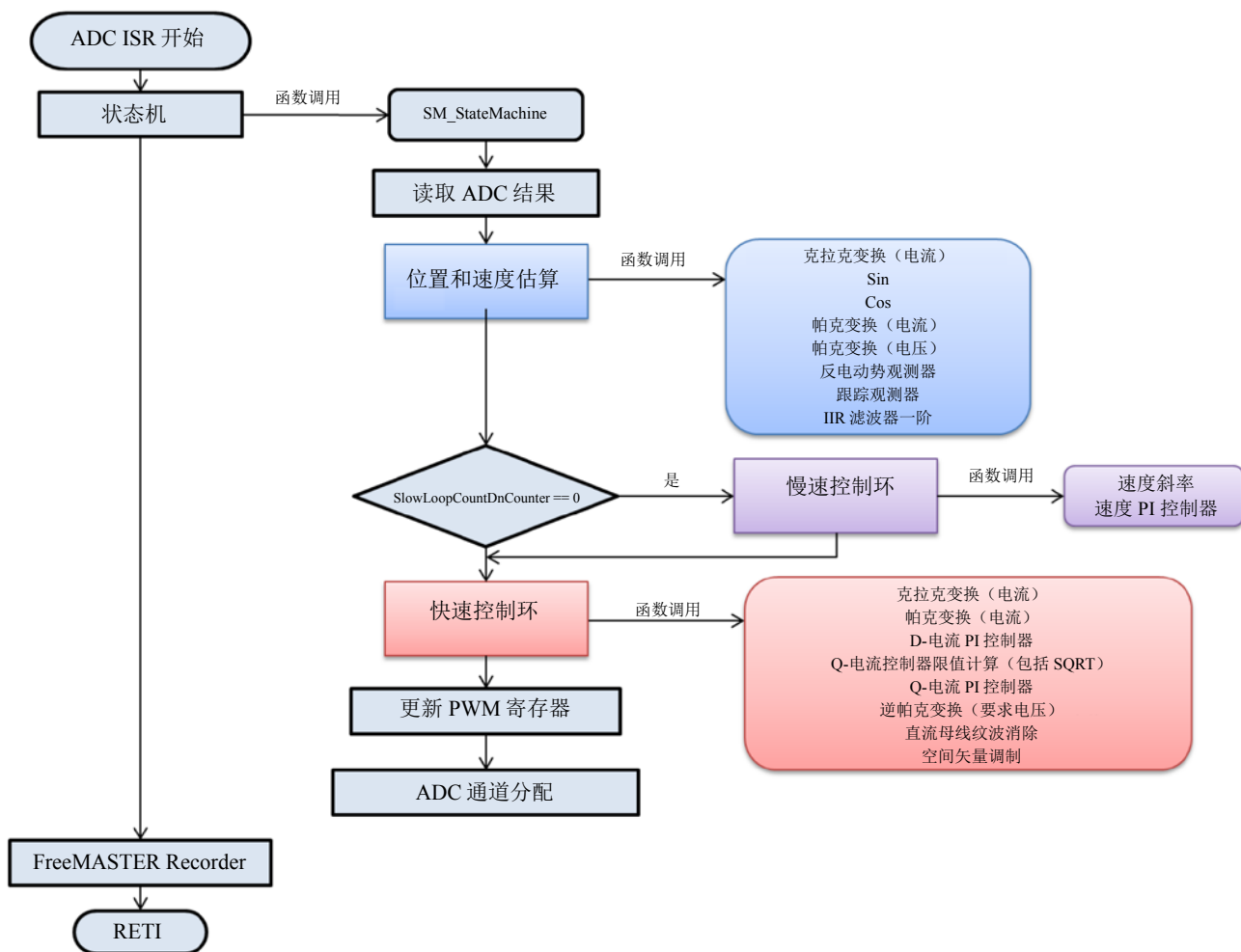
图 7. ADC ISR流程图
