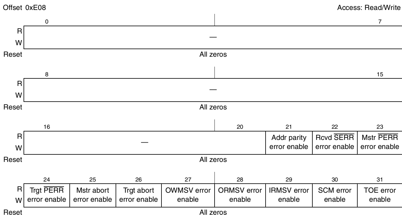
Figure 17-17. PCI Error Enable Register (ERR_EN)
