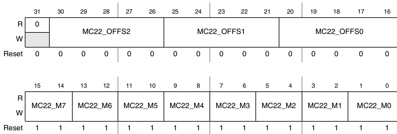
Figure 44-113. DI Display 2 Command Byte 2 Mapping Register (DI_DISP2_CB2_MAP)
