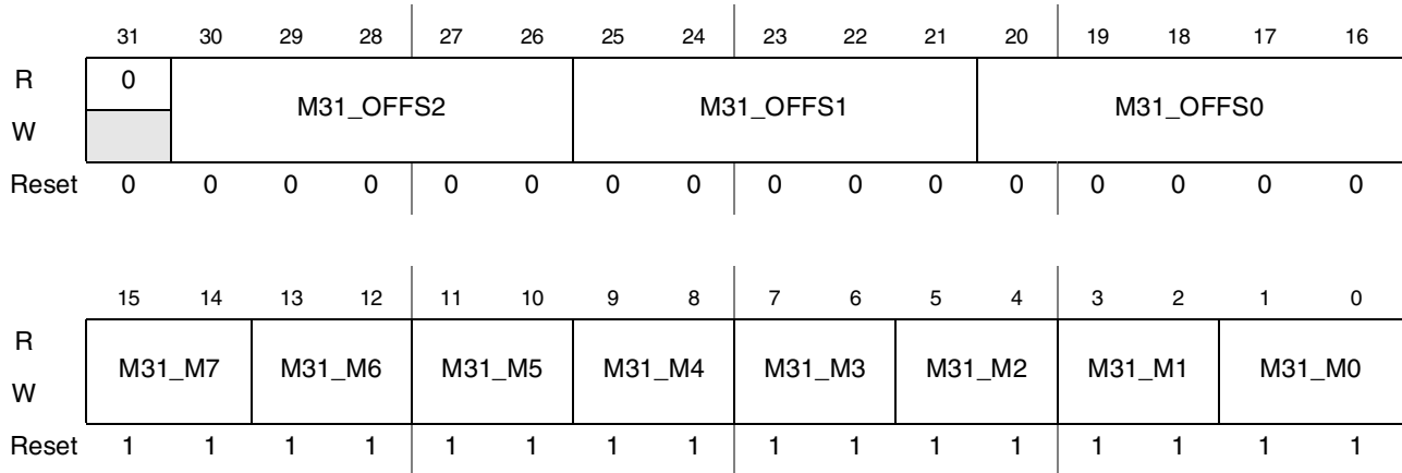
Figure 44-115. DI Display 3 Byte 1 Mapping Register (DI_DISP3_B1_MAP)
