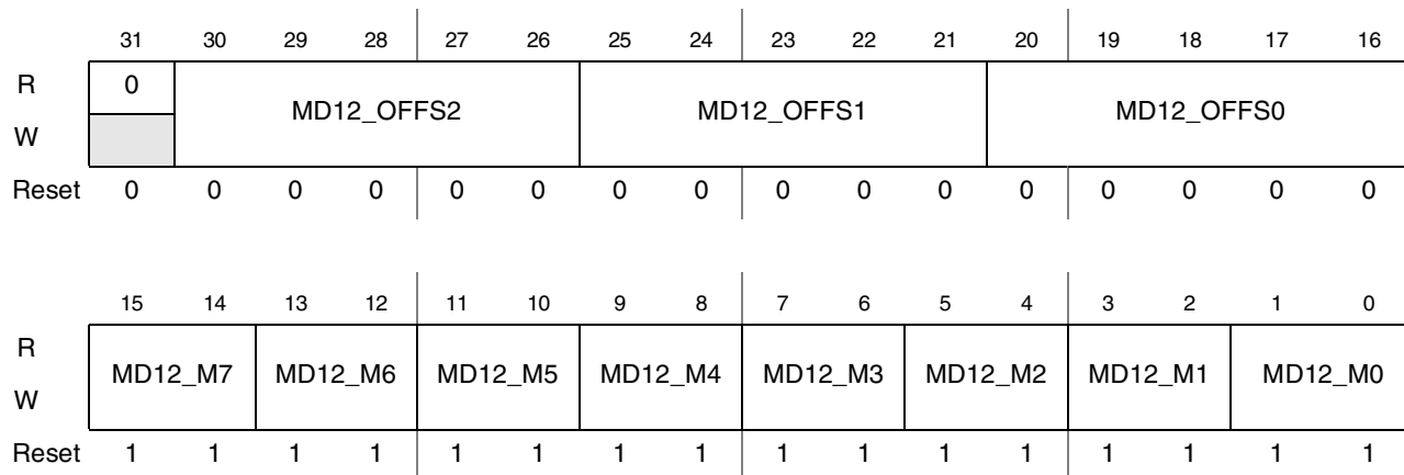
Figure 44-104. DI Display 1 Data Byte 2 Mapping Register (DI_DISP1_DB2_MAP)
