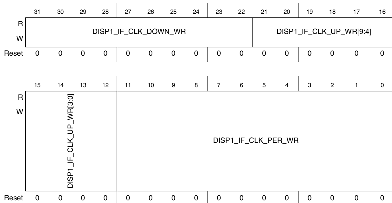
Figure 44-89. DI Display 1 Time Configuration Register 1 (DI_DISP1_TIME_CONF_1)
