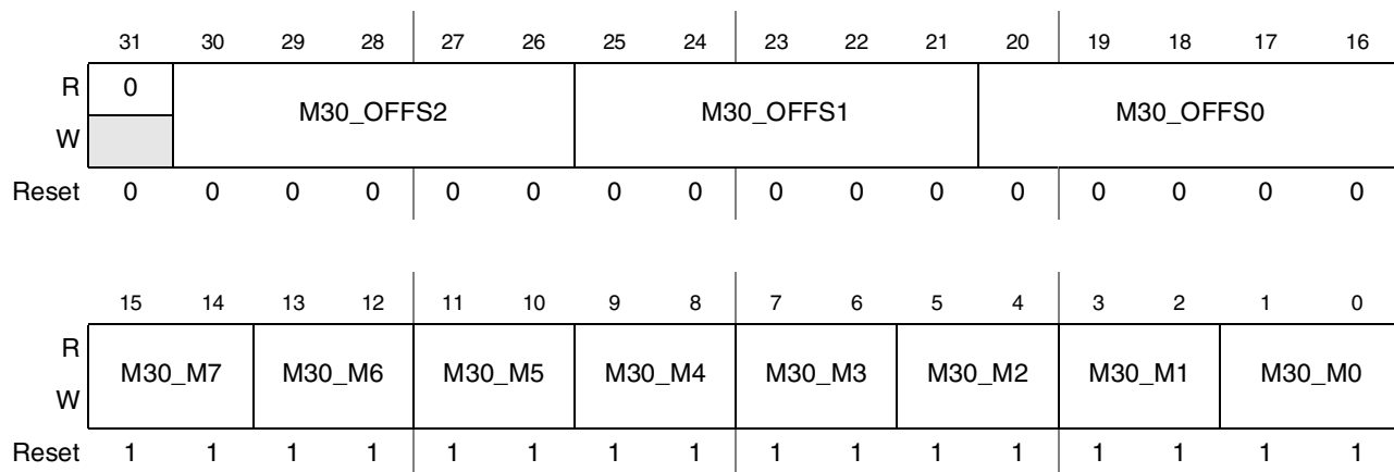
Figure 44-114. DI Display 3 Byte 0 Mapping Register (DI_DISP3_B0_MAP)
