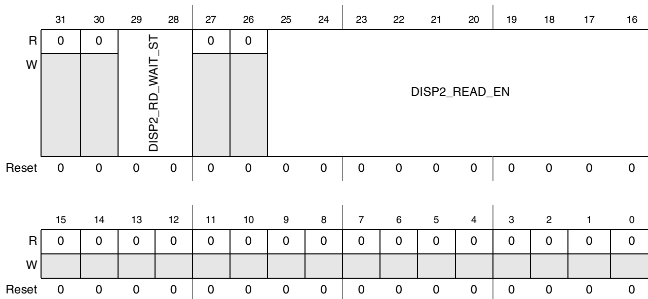
Figure 44-94. DI Display 2 Time Configuration Register 3 (DI_DISP2_TIME_CONF_3)
