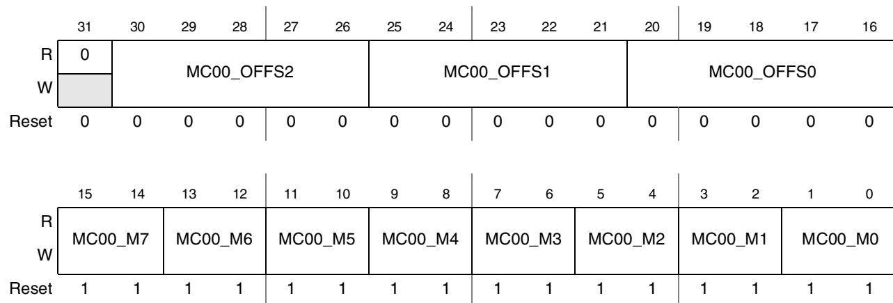
Figure 44-99. DI Display 0 Command Byte 0 Mapping Register (DI_DISP0_CB0_MAP)
