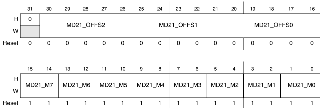
Figure 44-109. DI Display 2 Data Byte 1 Mapping Register (DI_DISP2_DB1_MAP)
