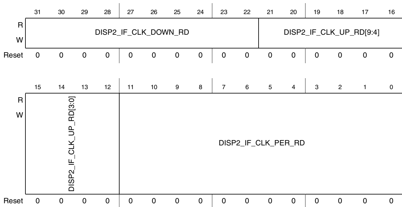
Figure 44-93. DI Display 2 Time Configuration Register 2 (DI_DISP2_TIME_CONF_2)
