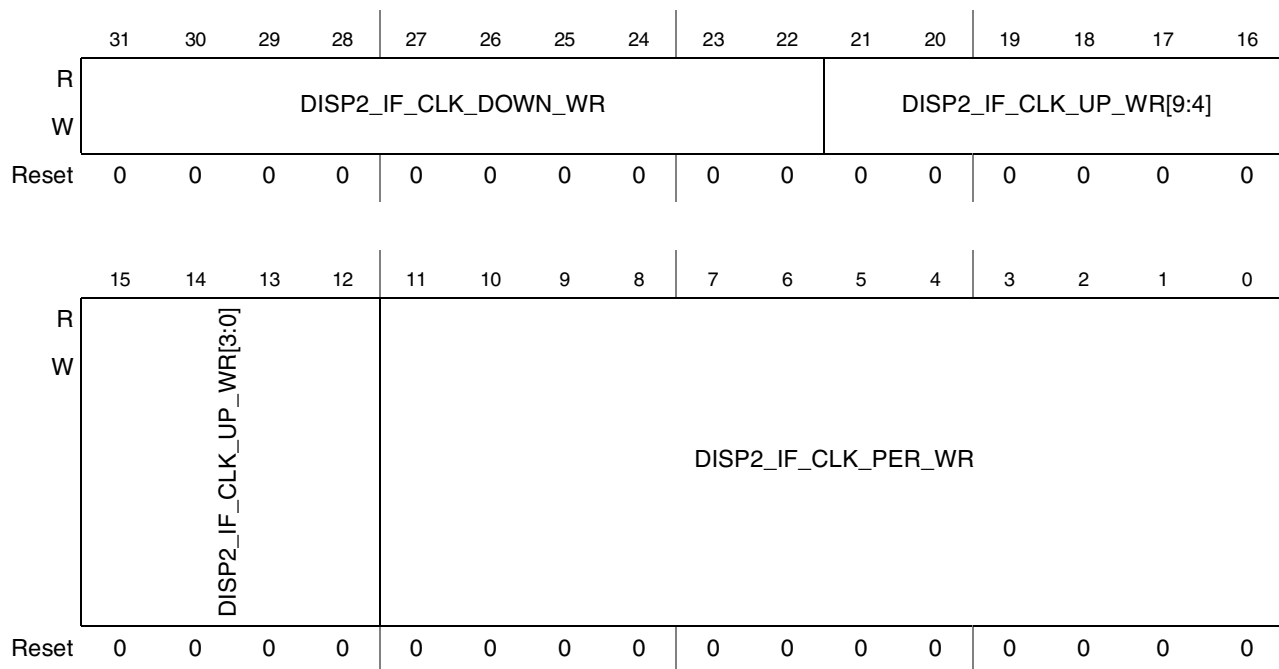
Figure 44-92. DI Display 2 Time Configuration Register 1 (DI_DISP2_TIME_CONF_1)
