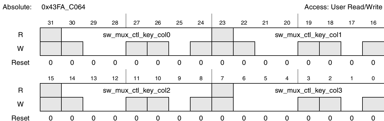
Figure 4-28. Register Description sw_mux_ctl_key_col0_key_col1_key_col2_key_col3
