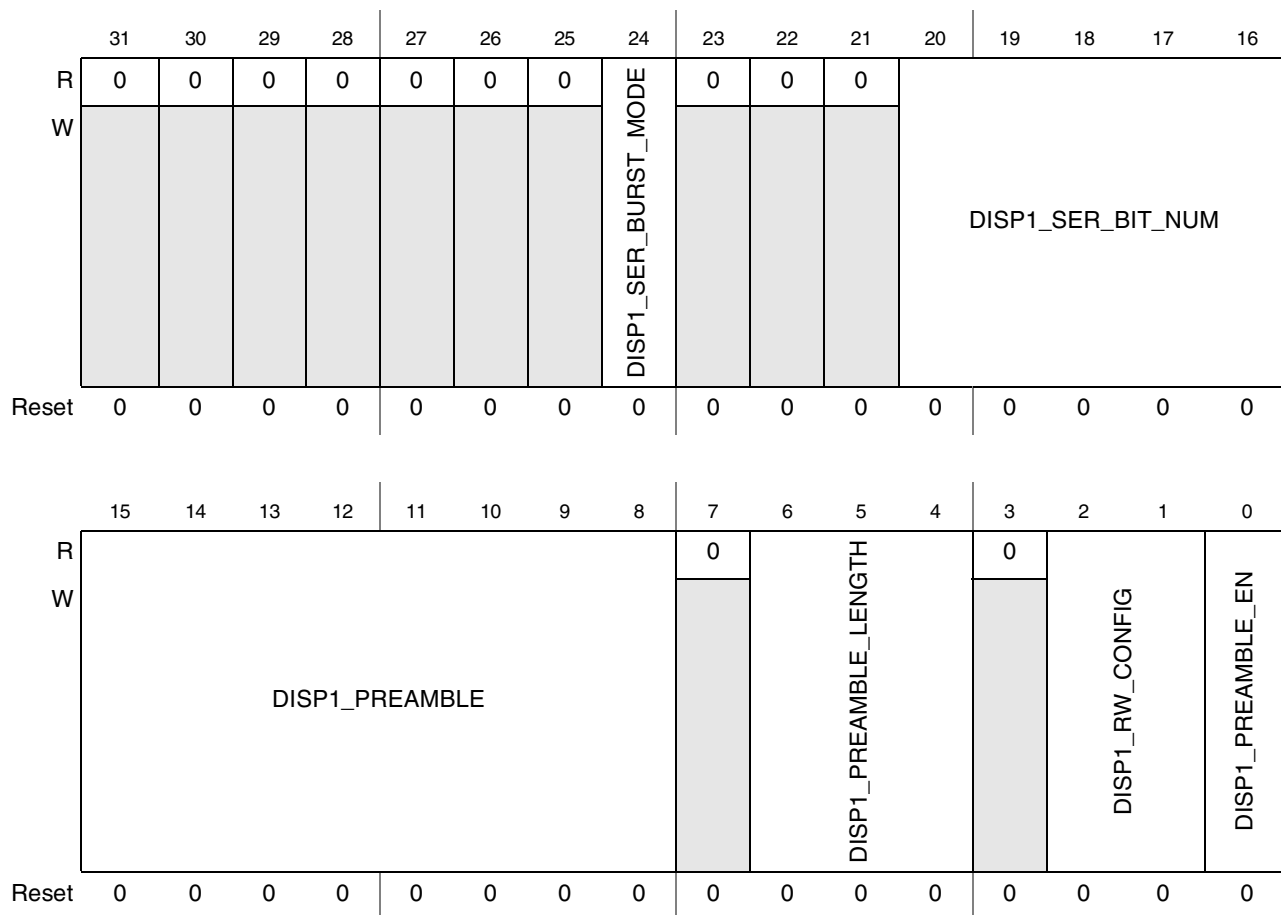
Figure 44-83. DI Serial Display 1 Configuration Register (DI_SER_DISP1_CONF)
