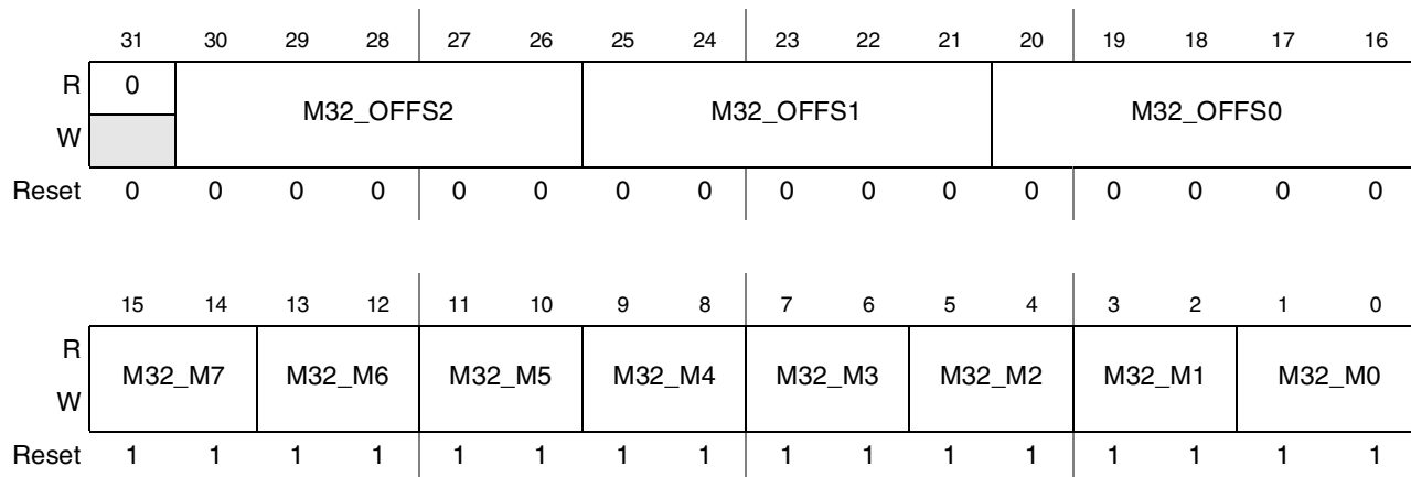
Figure 44-116. DI Display 3 Byte 2 Mapping Register (DI_DISP3_B2_MAP)
