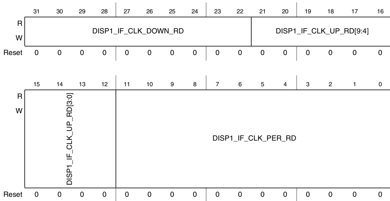
Figure 44-90. DI Display 1 Time Configuration Register 2 (DI_DISP1_TIME_CONF_2)
