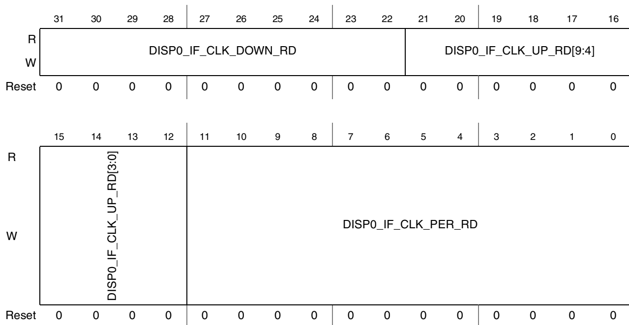
Figure 44-87. DI Display 0 Time Configuration Register 2 (DI_DISP0_TIME_CONF_2)
