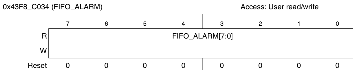
Figure 23-44. FIFO_ALARM Register
