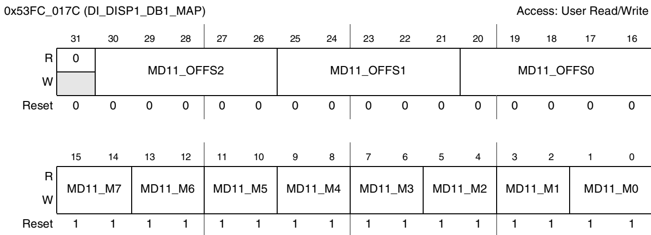
Figure 44-103. DI Display 1 Data Byte 1 Mapping Register (DI_DISP1_DB1_MAP)
