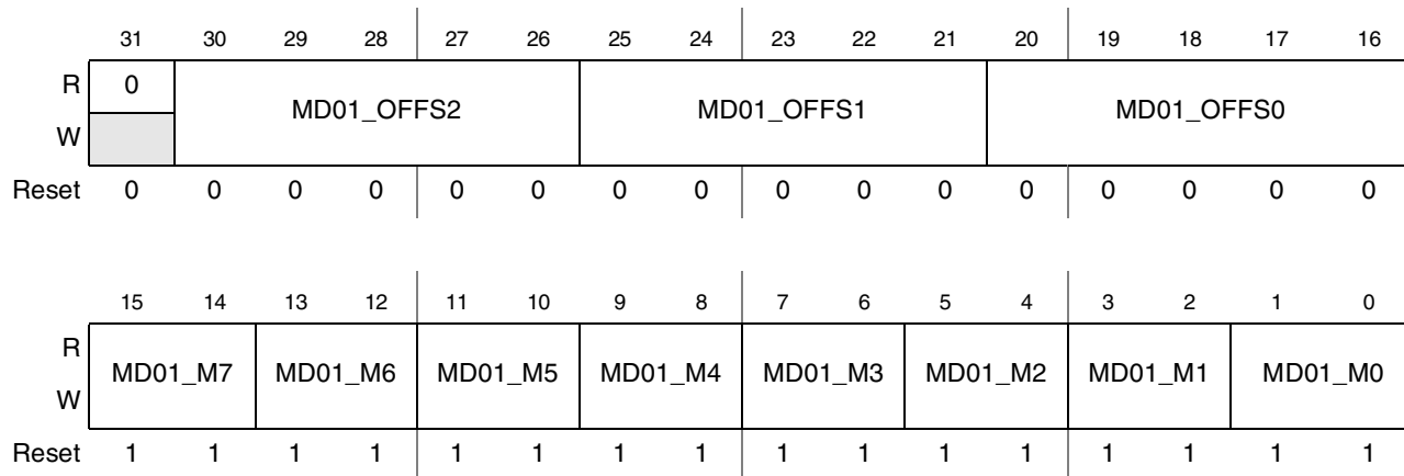
Figure 44-97. DI Display 0 Data Byte 1 Mapping Register (DI_DISP0_DB1_MAP)
