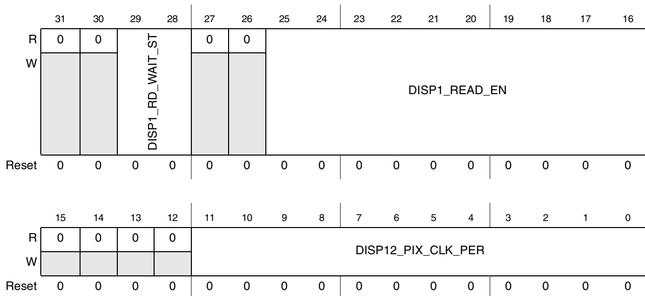
Figure 44-91. DI Display 1 Time Configuration Register 3 (DI_DISP1_TIME_CONF_3)
