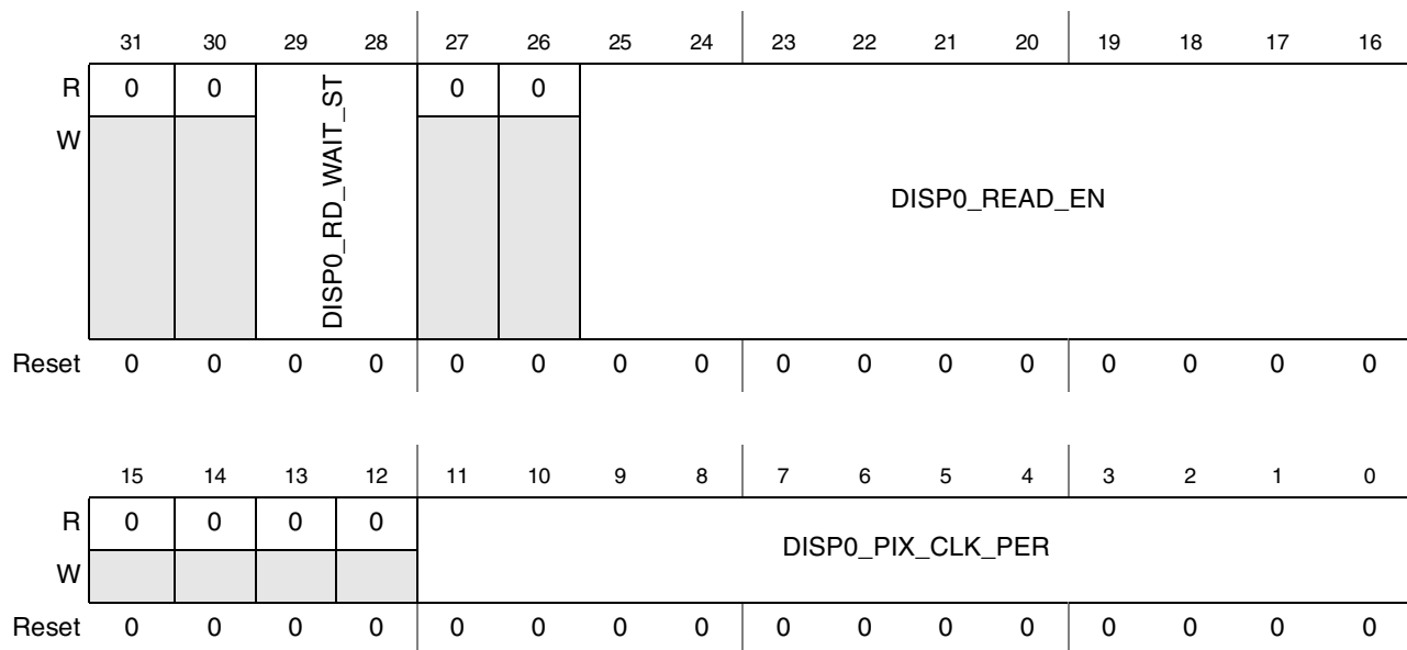
Figure 44-88. DI Display 0 Time Configuration Register 3 (DI_DISP0_TIME_CONF_3)
