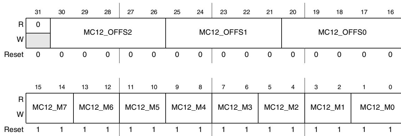
Figure 44-107. DI Display 1 Command Byte 2 Mapping Register (DI_DISP1_CB2_MAP)
