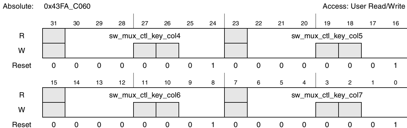
Figure 4-27. Register Description sw_mux_ctl_key_col4_key_col5_key_col6_key_col7
