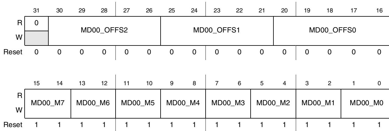
Figure 44-96. DI Display 3 Data Byte 0 Mapping Register (DI_DISP0_DB0_MAP)
