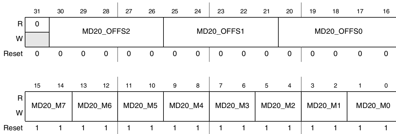
Figure 44-108. DI Display 2 Data Byte 0 Mapping Register (DI_DISP2_DB0_MAP)
