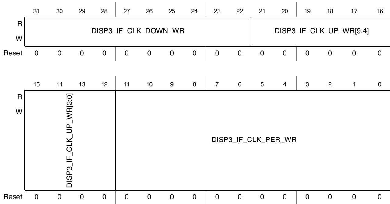
Figure 44-95. DI Display 3 Time Configuration Register (DI_DISP3_TIME_CONF)
