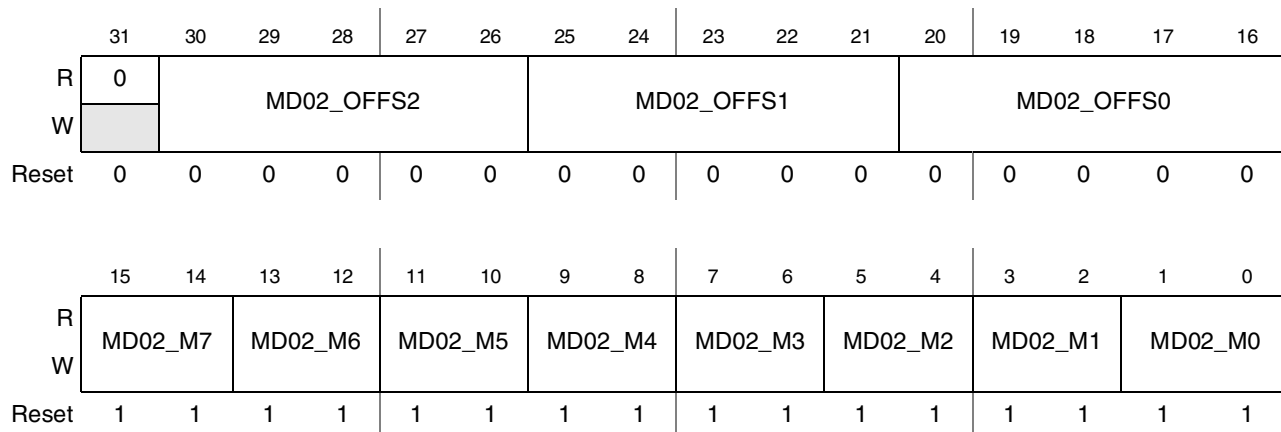
Figure 44-98. DI Display 0 Data Byte 2 Mapping Register (DI_DISP0_DB2_MAP)
